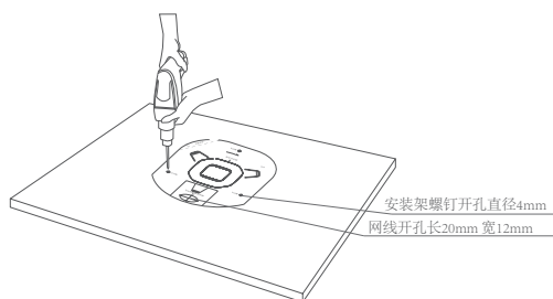
图3-3 钻孔示意图
